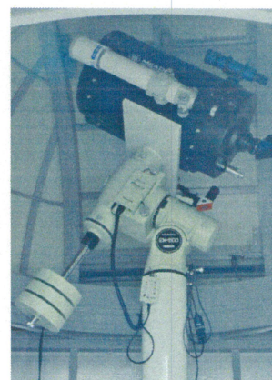
シュミットカセグレン式天体望遠鏡
